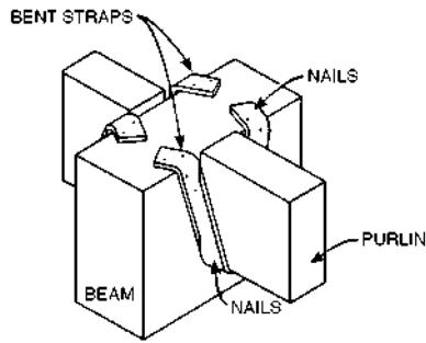
Fig. 27. Bent strap purlin hanger
