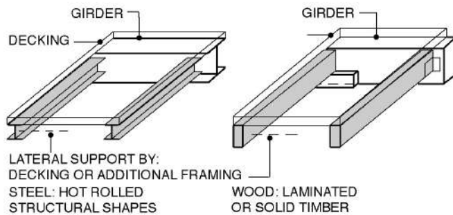
Fig. 23. Beams
