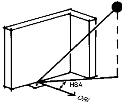
Fig.10. Horizontal shadow angle (HSA)
