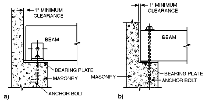
Fig. 29. Beam anchorage
