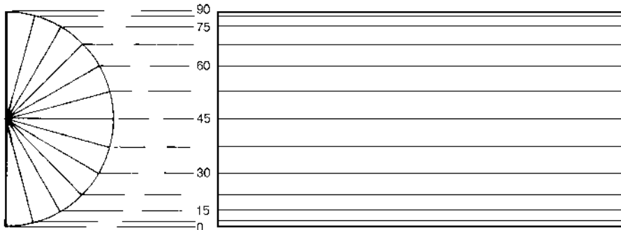
Fig. 20. Waldram projection
