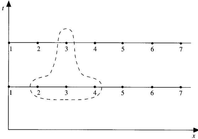
FIG. 4.7 An explicit finite-difference module.
