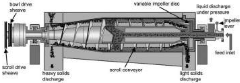
FIG. 18-160 Sortercanter centrifuge. (Flottweg Separation Technology.)
