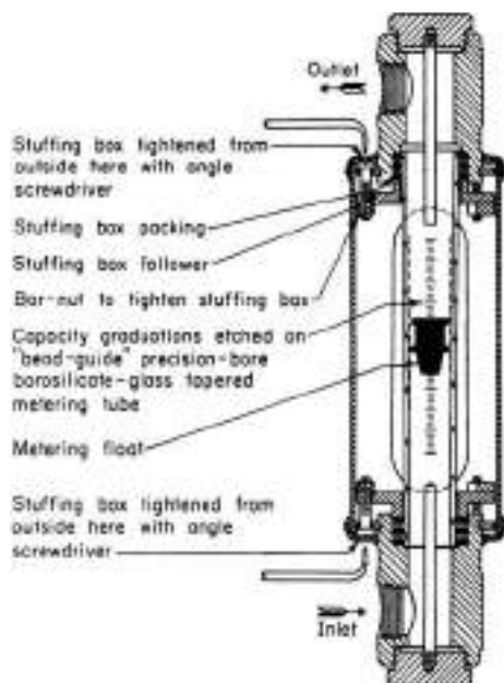
FIG. 10-20 Rotameter.
